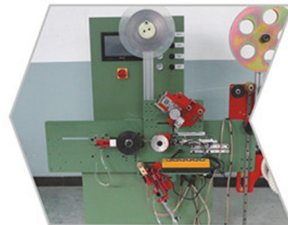
自动缠绕设备
